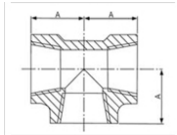
Tee
