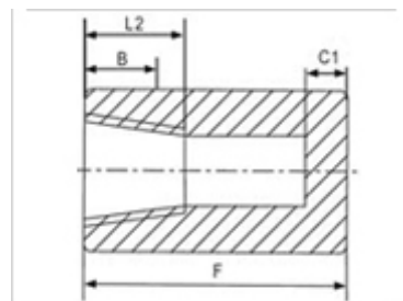
Cap
